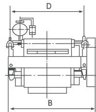
外形尺寸图
